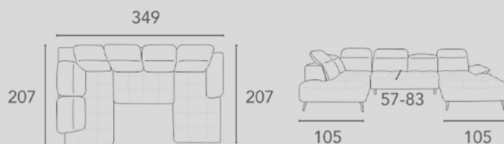
Zostava U L / P Motorové prehĺbenie sedu
